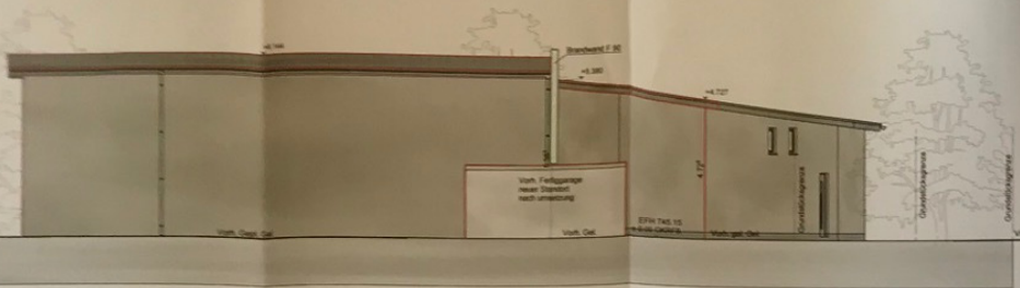
Nordansicht M 1:100
