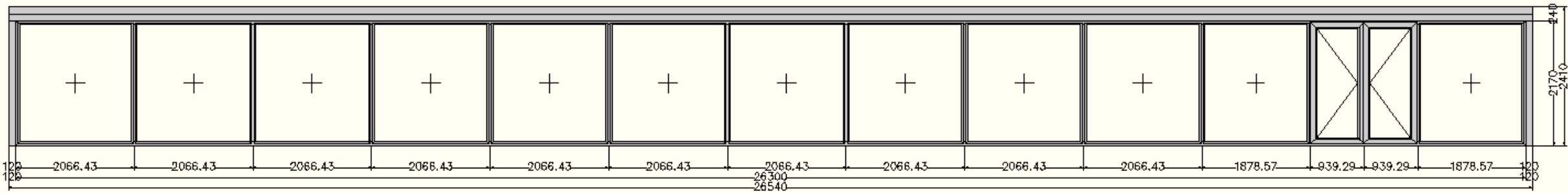
Ansicht von innen (Maßstab 1:50)
