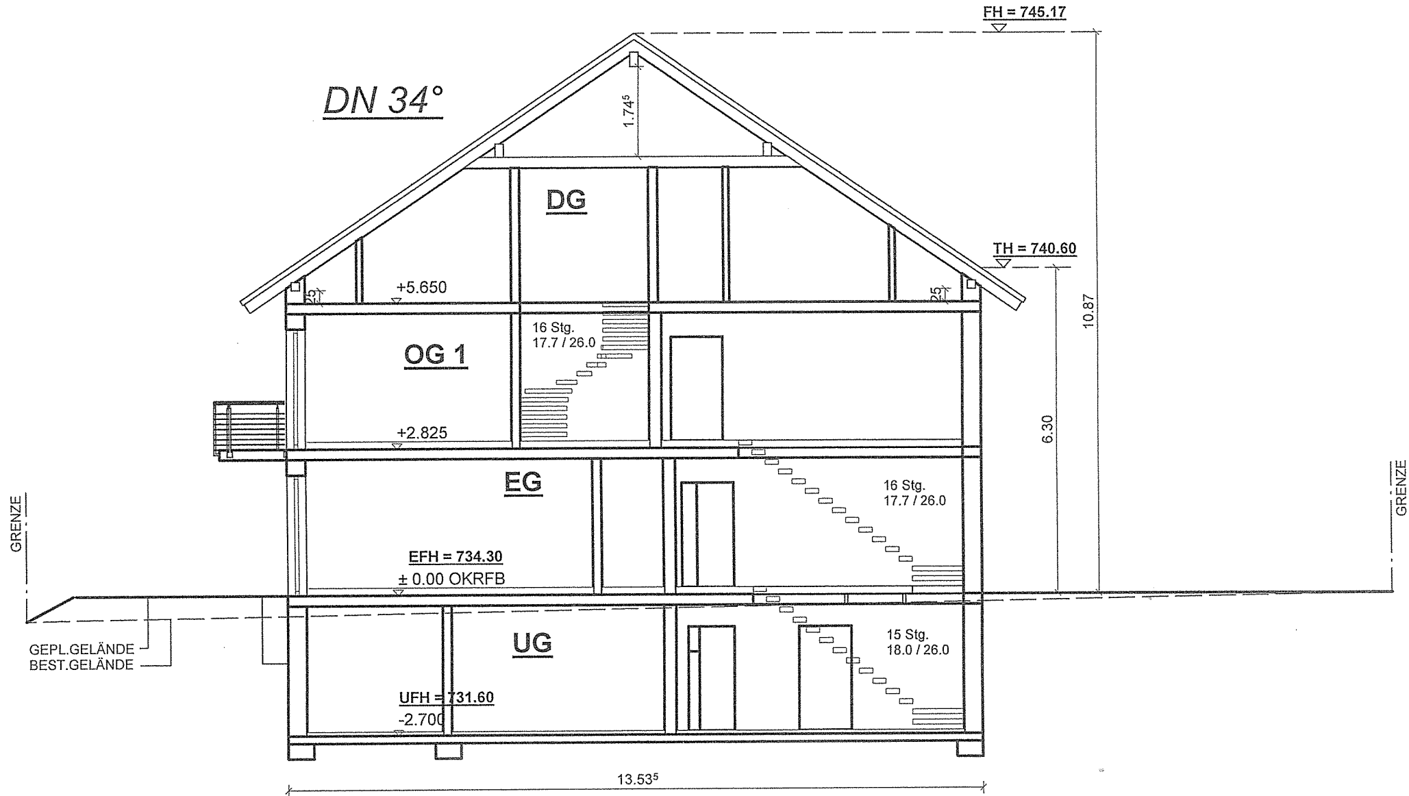
SCHNITT A-A
