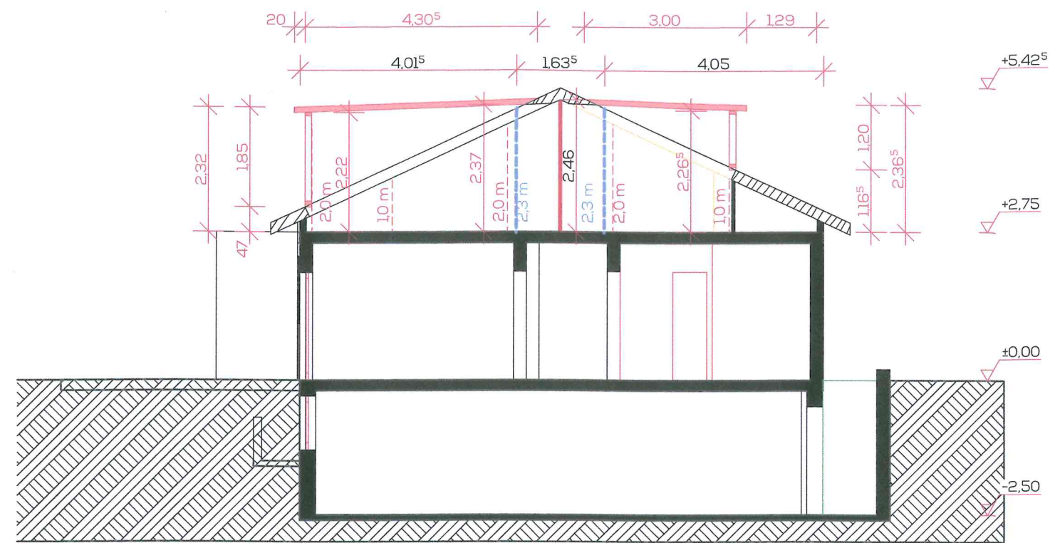
Schnitt 01-01
