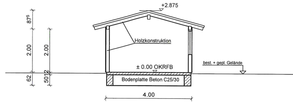
Schnitt
