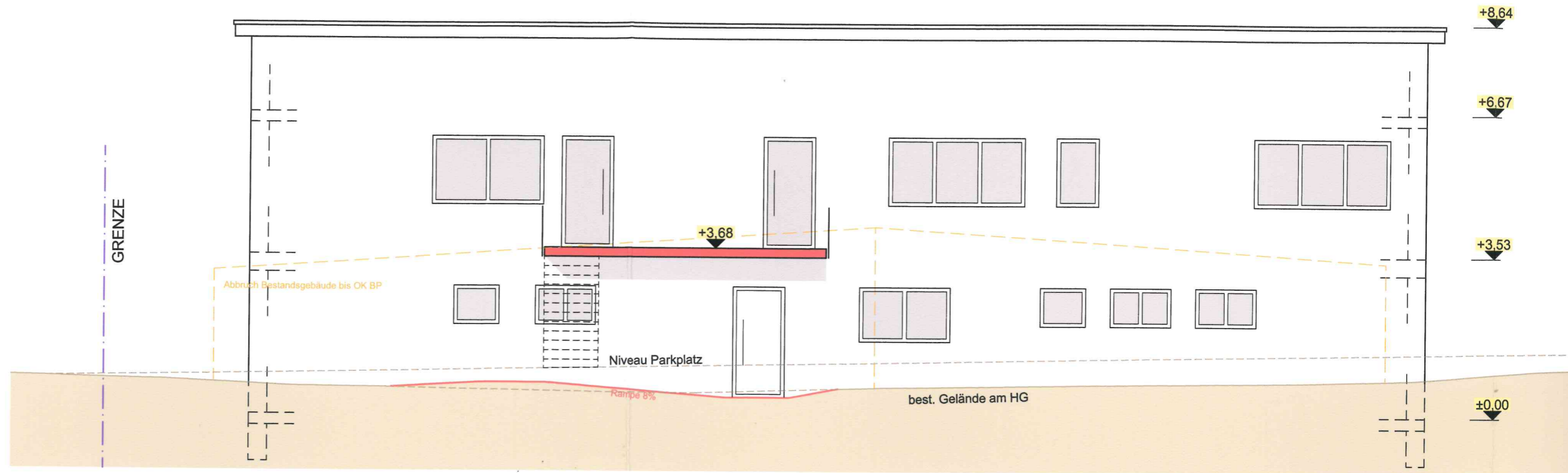
ANSICHT NORD-WEST
