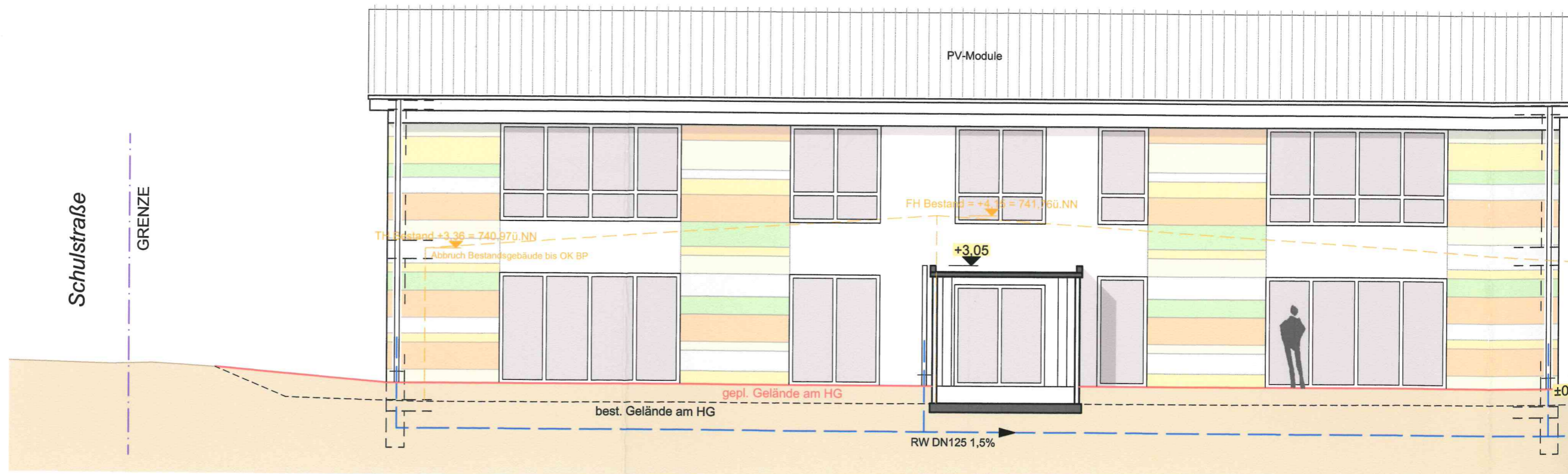
ANSICHT SÜD-OST
