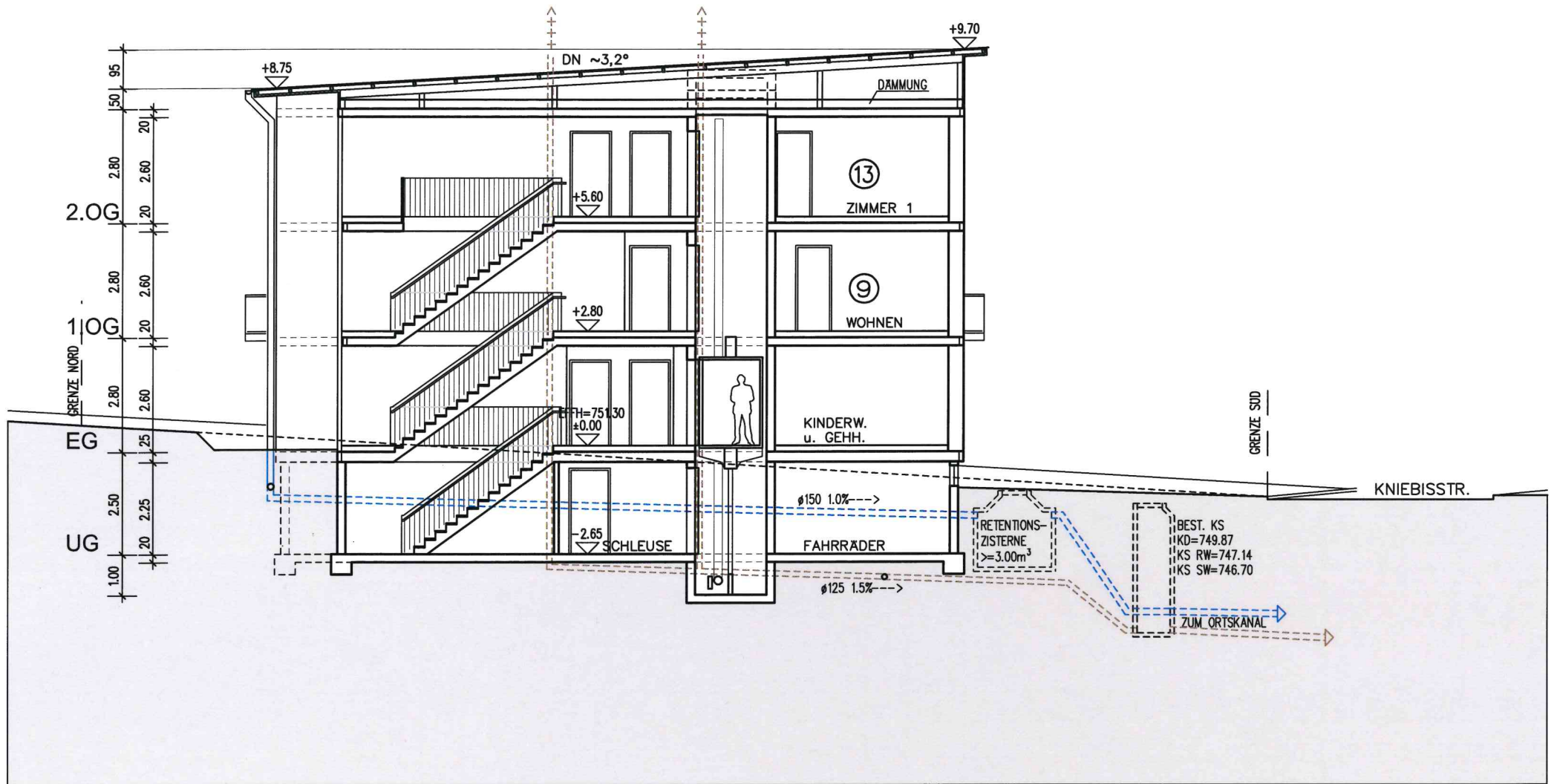
Schnitt A
