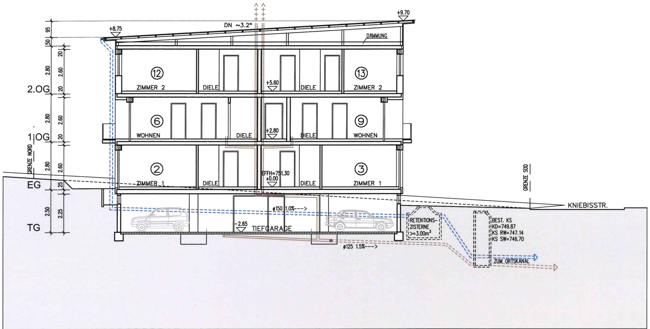
Schnitt B
