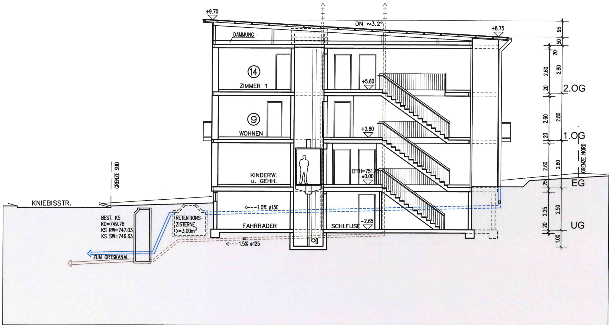
Schnitt A
