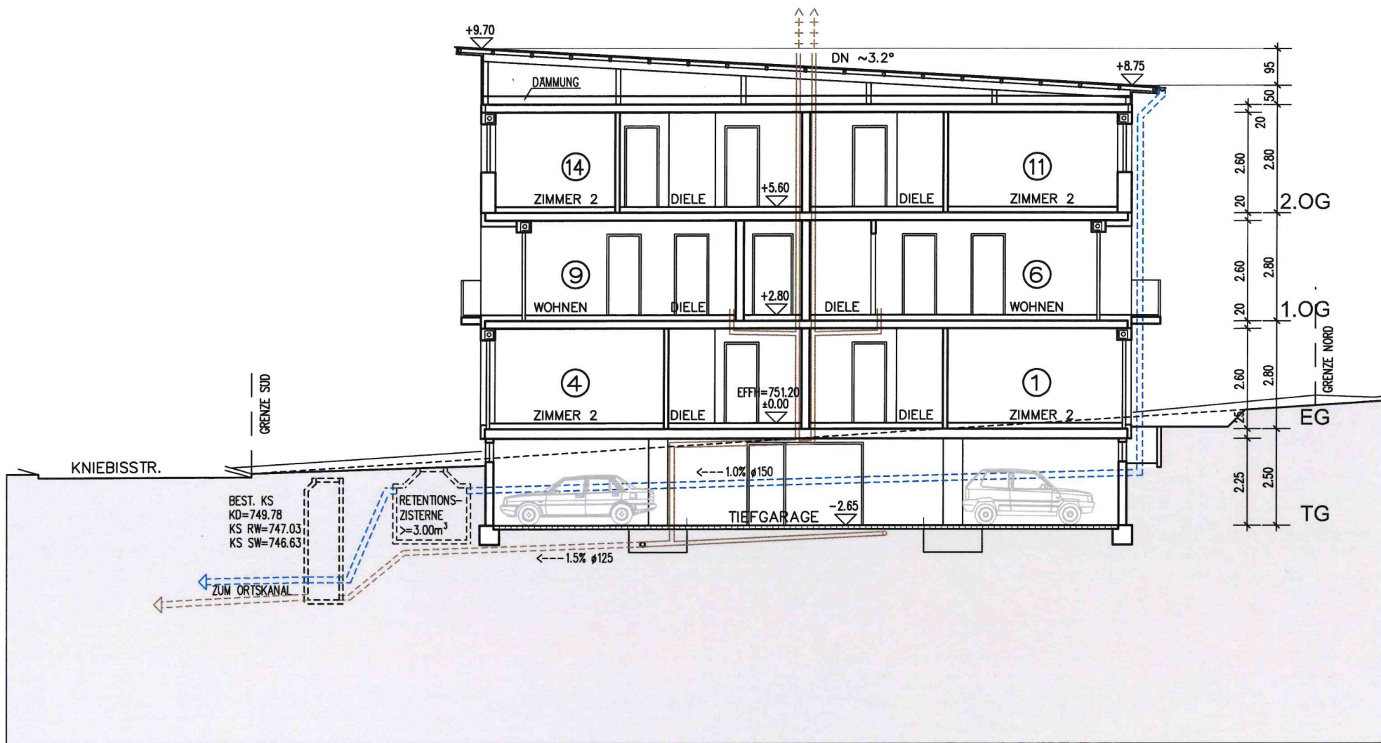
Schnitt B
