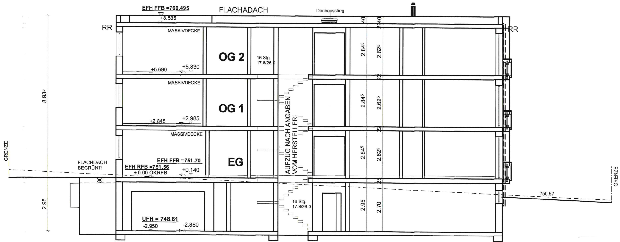
SCHNITT A-A
