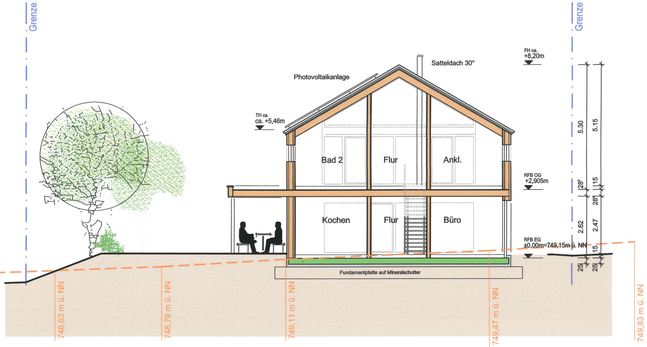
SCHNITT A-A M 1:100
