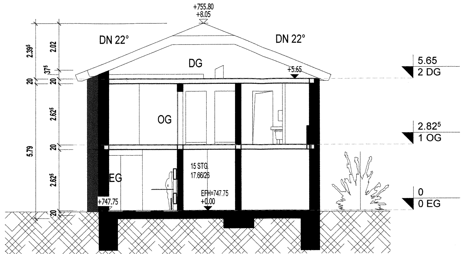
SCHNITT B
