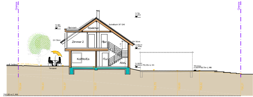
SCHNITT A-A M 1:100
